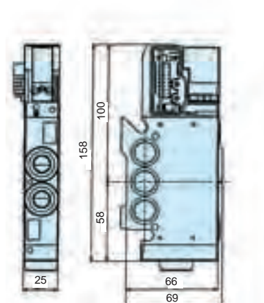
Distributeurs 5/2 monostables
