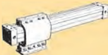
Simple chariot inversé avec plateau articulé
