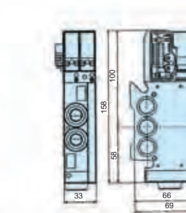
Distributeurs 5/2 bistables - 2x3/2 - 5/3
